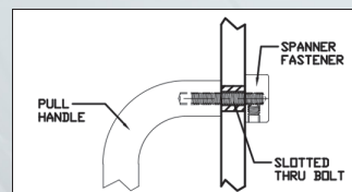
Glass Door Thru Bolt Type 15HD
