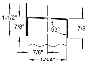
A548B ● BEVELED EDGE ● NON-MORTISED
