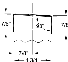
A528BM ● BEVELED EDGE ● MORTISED
