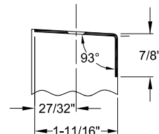
A528BM ● BEVELED EDGE ● MORTISED
