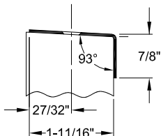
A528B ● BEVELED EDGE ● NON-MORTISED
