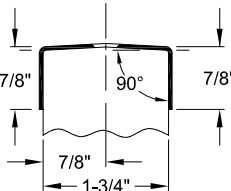
A538R ● RADIUS EDGE ● NON-MORTISED
