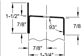
A548BM ● BEVELED EDGE ● MORTISED
