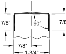
A538RM ● RADIUS EDGE ● MORTISED
