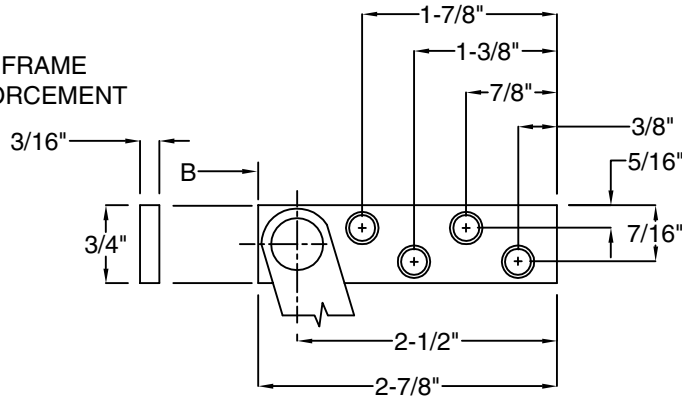
JAMB BRACKET
